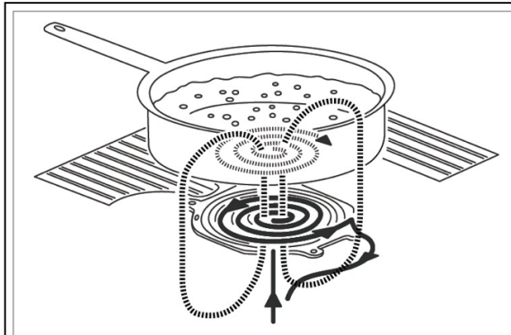
Principio di funzionamento e struttura schematica di una cucina a induzione
